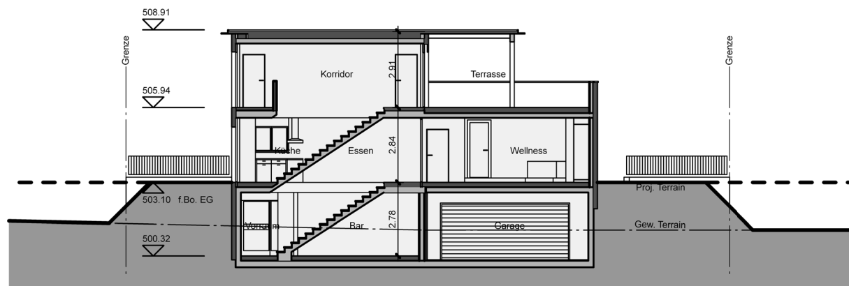
Querschnitt A-A
