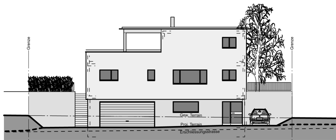
Ostfassade
