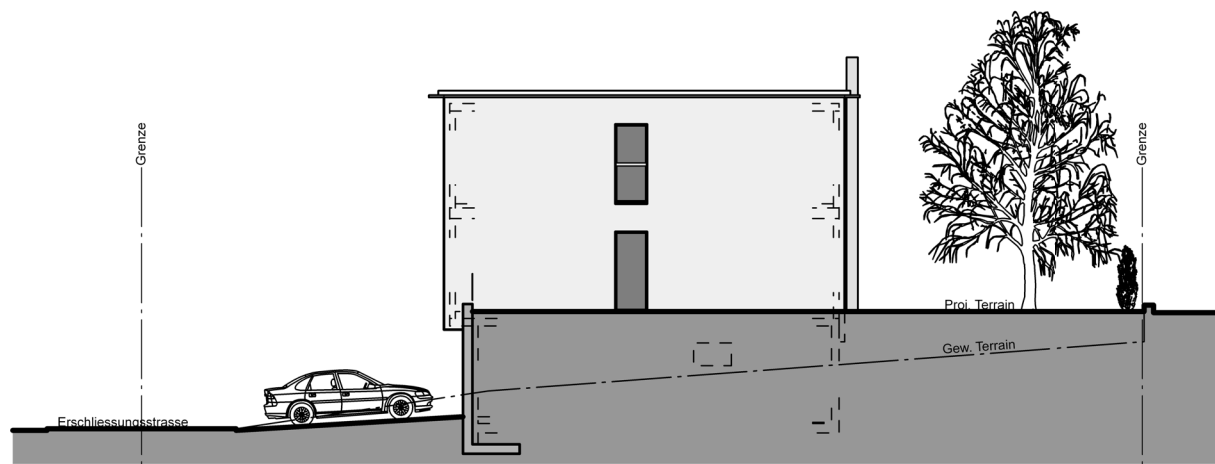
Nordfassade
