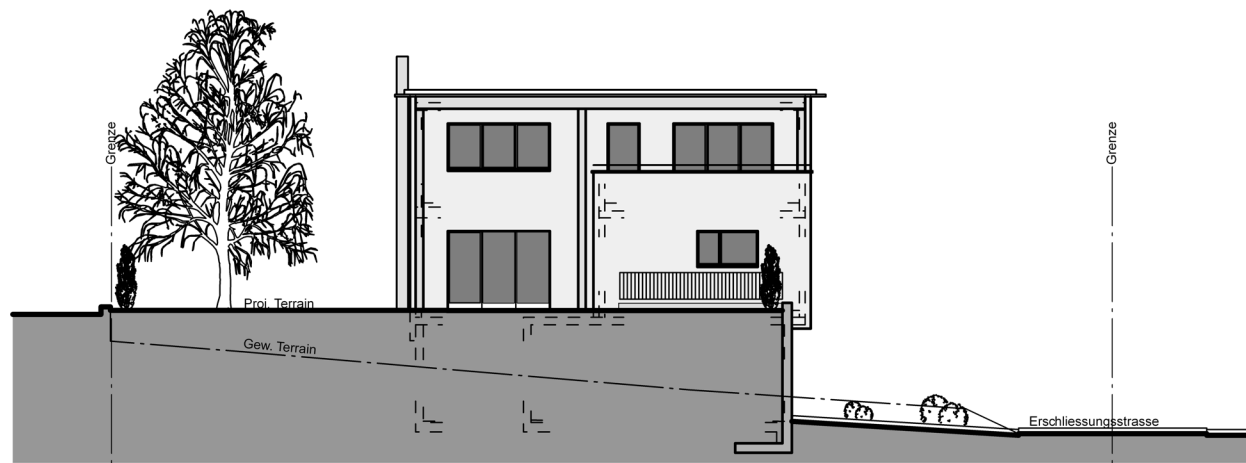
Südfassade
